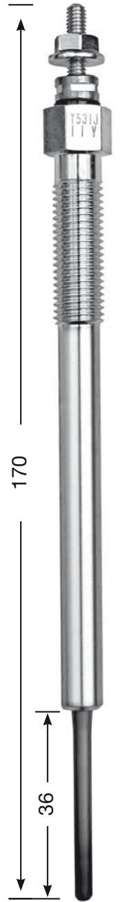
Y-531 J M 10 x 1.25 12 Hex 11 V DP 44
