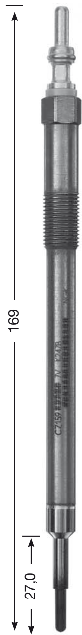
CZ 159 M 10 x 1.0 10 Hex 7 V DP 84
